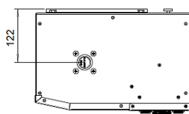
LÄMMITYSPIIRIN LIITÄNNÄT 3/4" Ulkokierre
