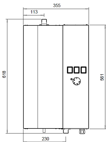
LÄMMITYSPIIRIN LIITÄNNÄT 3/4" Ulkokierre
